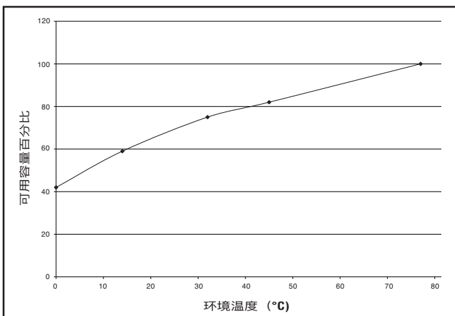
电池容量与工作温度
